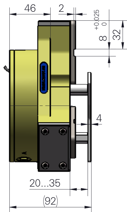
带推料装置图
