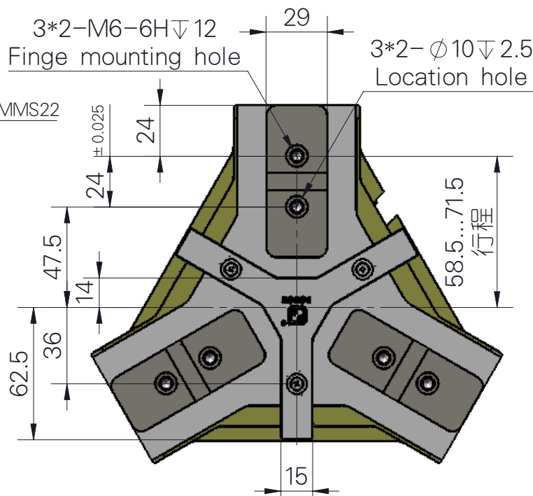
带推料装置图
