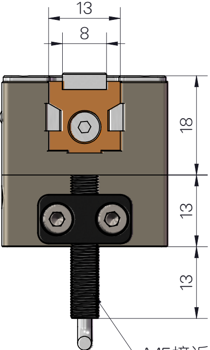
M5接近开关
